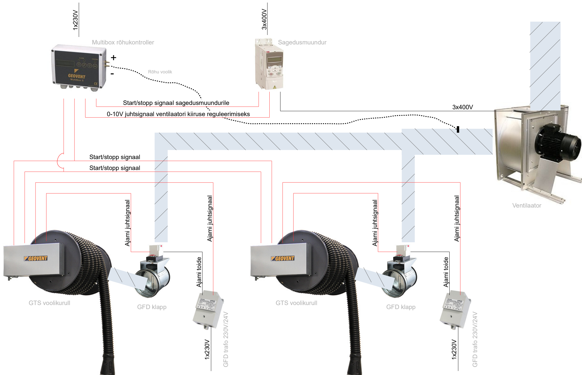
Põhimõtteline ühendusskeem – GTS voolikurullid + ventilaator + röhukontroller + sagedusmuundur + GFD sulgklapid
