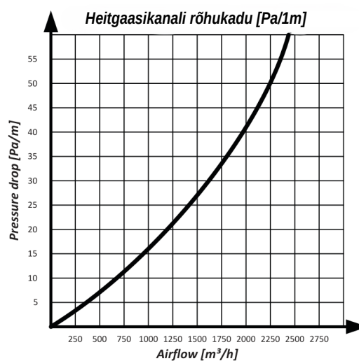
Graafik 2 – Rõhukao graafik heitgaasikanali, käru ja vooliku jaoks
