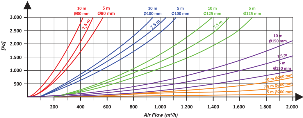
Graafik 1 – Õhuhulga ja rõhukao graafik GTE ja GTS voolikurullide jaoks
